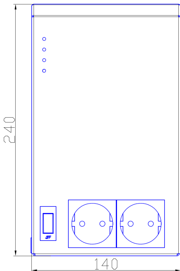
а) ИнСтаб 500
