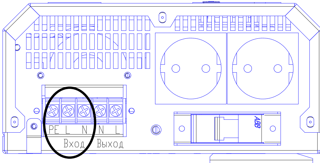
Рисунок 3.2 – Стабилизатор ИнСтаб 3500.
