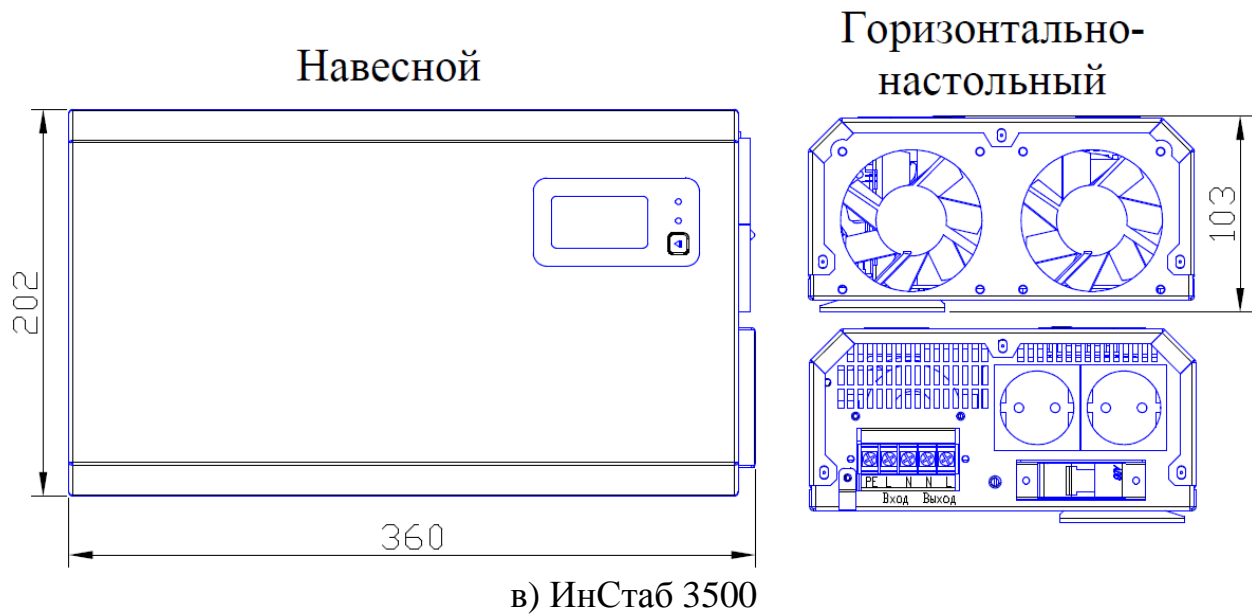
Рисунок 1.2. – Габаритные размеры стабилизатора Штиль и рекомендуемые варианты установки а) ИнСтаб 500; б) ИнСтаб 1000; ИнСтаб 1500; в) ИнСтаб 3500
